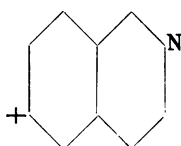
Brönnersche ( \beta ) Säure.
